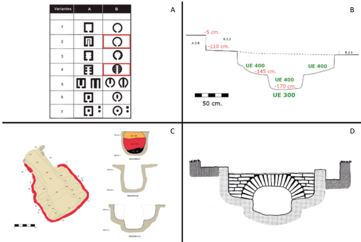
Fig. 11. A. Tipología de hornos ibéricos de Broncano y Coll (1988), con indicación de las tipologías B2 y B4. B. Perfil final de la hoya excavada en el alfar vacceo de Tordehumos. C. Perfil del horno medieval 1 de El Casetón de la Era (Crespo, 2014: 407, fig. 5). D. Perfil y reconstrucción del horno hispano-romano de Relea (Juan y Pérez, 1987: 666, fig. 3).
