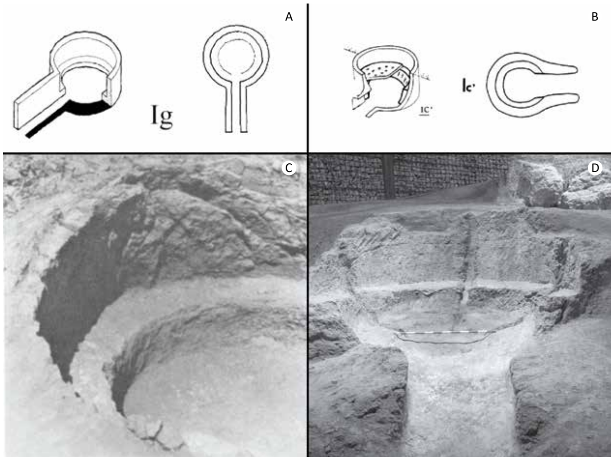
Fig. 10. A. Tipología Ig para los hornos cerámicos griegos de la Antigüedad propuesta por E. Hasaki (2002: 158, 501, lám. III.4). B. Tipología Ic' para los hornos galo-romanos propuesta por Le Ny (1988: 39-65; fig. 22a y 23). C. Horno cerámico de Palaikastro (Creta) (Davaras, 1980: lám. 7, C). D. Horno cerámico romano n.º 3 de la Fornaca (Vilassar de Dalt, Barcelona) (Roselló, Gironés y Gamarra, 2006-2007: 198, fig. 3).
